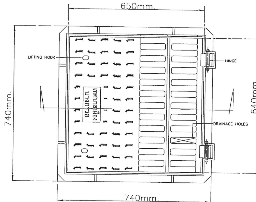
แปลน ฝาบ่อ มาตรฐาน 1:7.5
