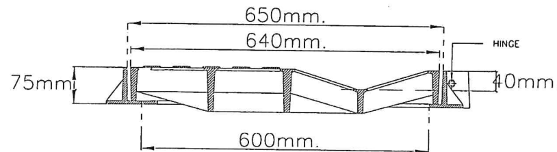
รูปตัด มาตรฐาน 1:7.5
